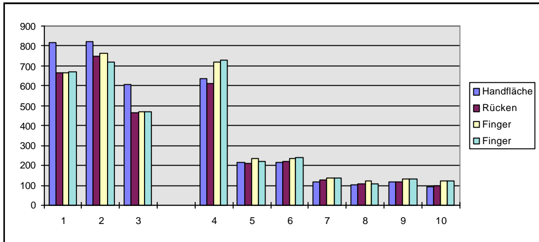
Abb. 3: Streuung der Materialstärke bei 10 zufällig ausgewählten Handschuhen Alle Ergebnisse in µm bzw. in Prozent Standardabweichung Handschuh 1 bis 3 mit profilierter Handfläche
