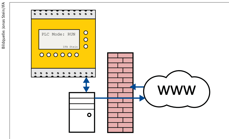
Abbildung 3: Die Sicherheitssteuerung ist hier mit einem Rechner verbunden. Beide befinden sich innerhalb einer demilitarisierten Zone und sind durch eine Firewall geschützt. Der Rechner erhielt jedoch über eine E-Mail eine Schadsoftware, mit der ein Tunnel durch die Firewall geöffnet werden konnte. Über den kompromittierten Rechner kann nun die Steuerung leicht angegriffen werden.
